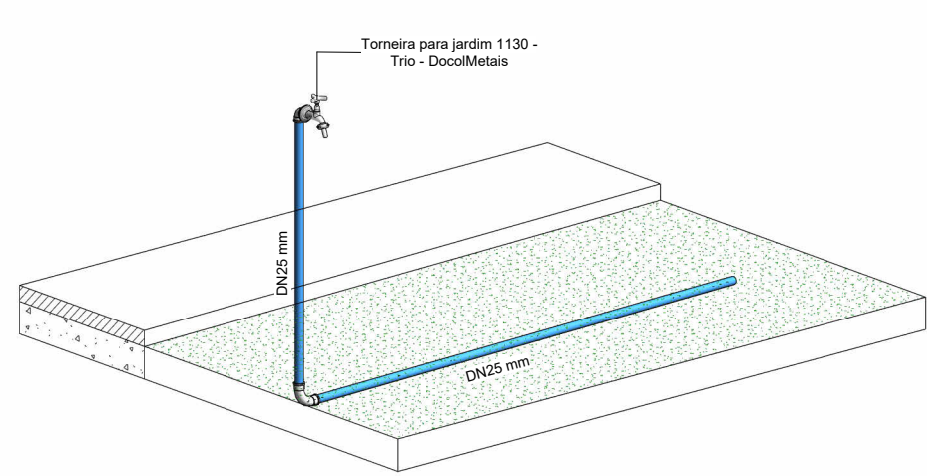
3 DETALHE 3D TORNEIRAS 02 ESCALA
