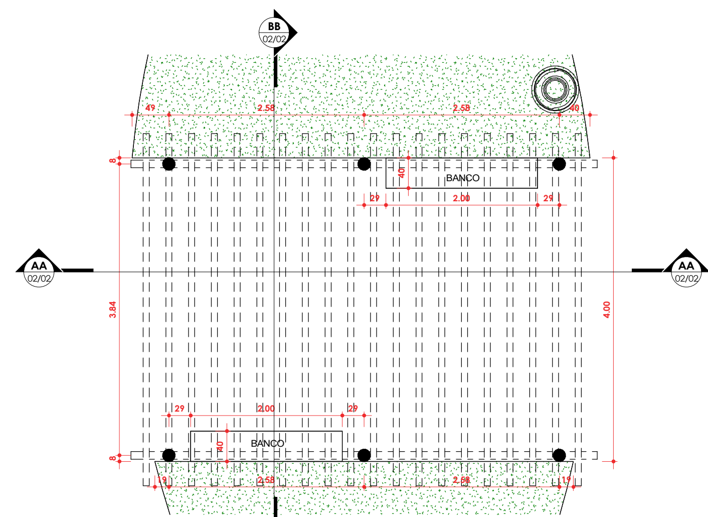
3 PLANTA BAIXA - CARAMANCHÃO 1 : 50
