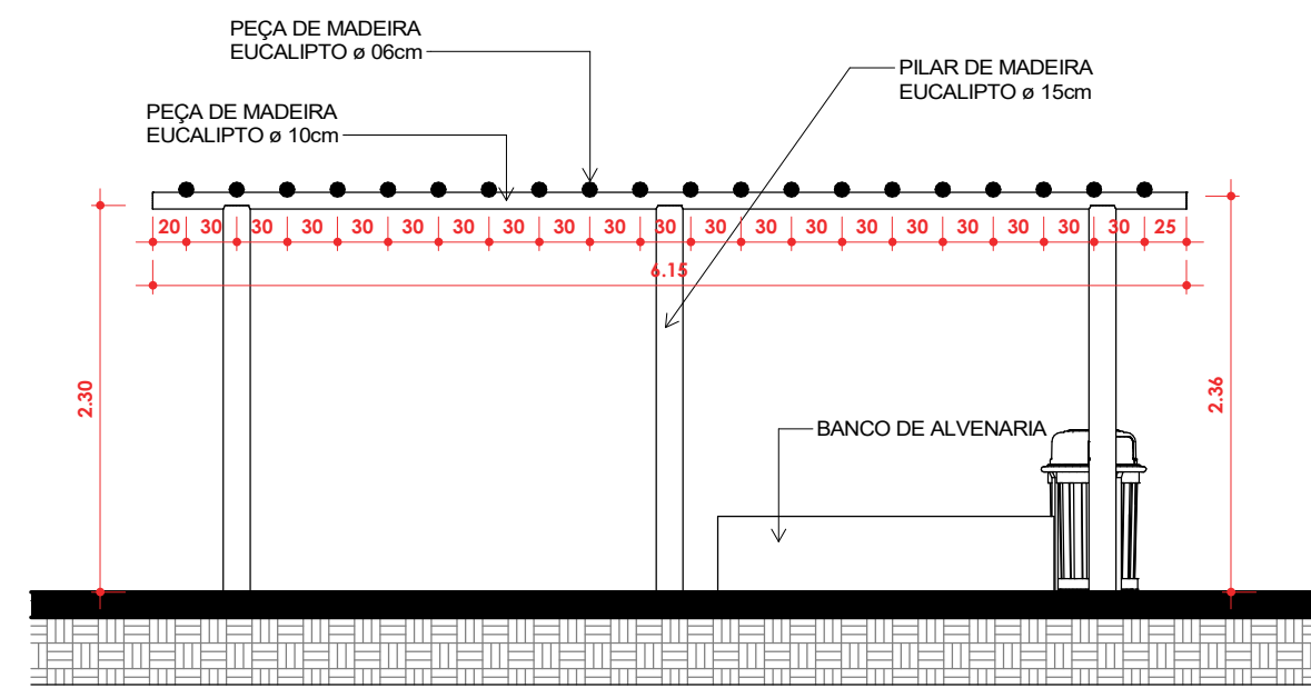
4 CORTE - AA 1 : 50
