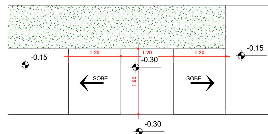
7 DET. RAMPA 1 : 50
