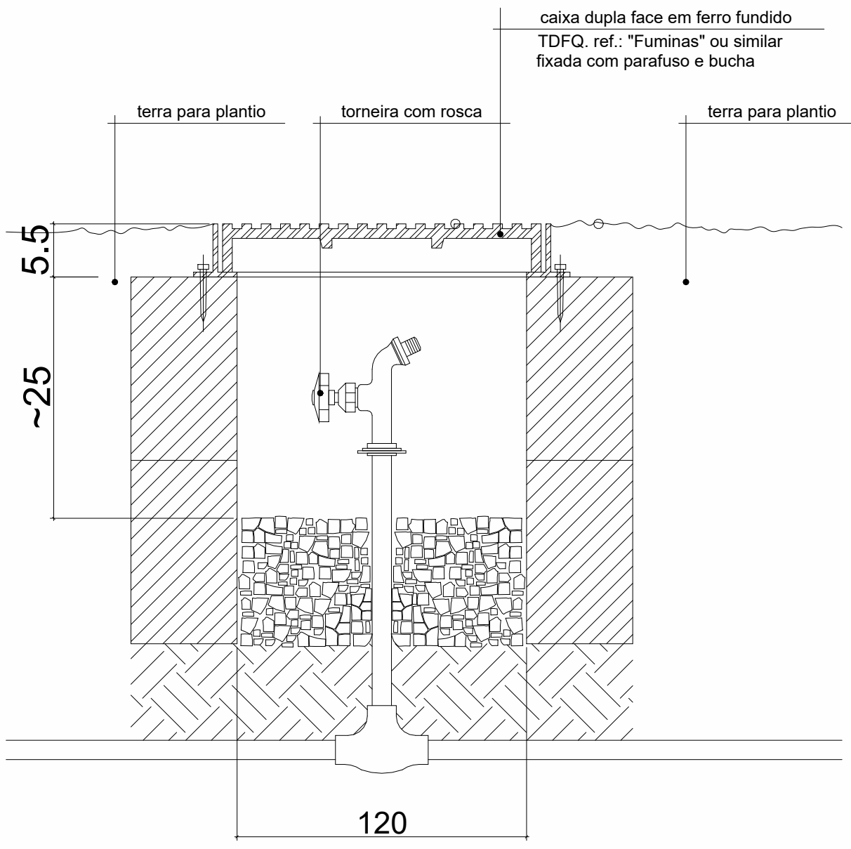
TORNEIRAS - JARDIM 1/50 ESCALA
