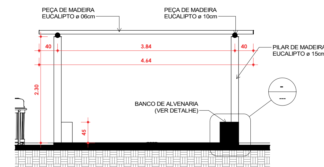
5 CORTE - BB 1 : 50
